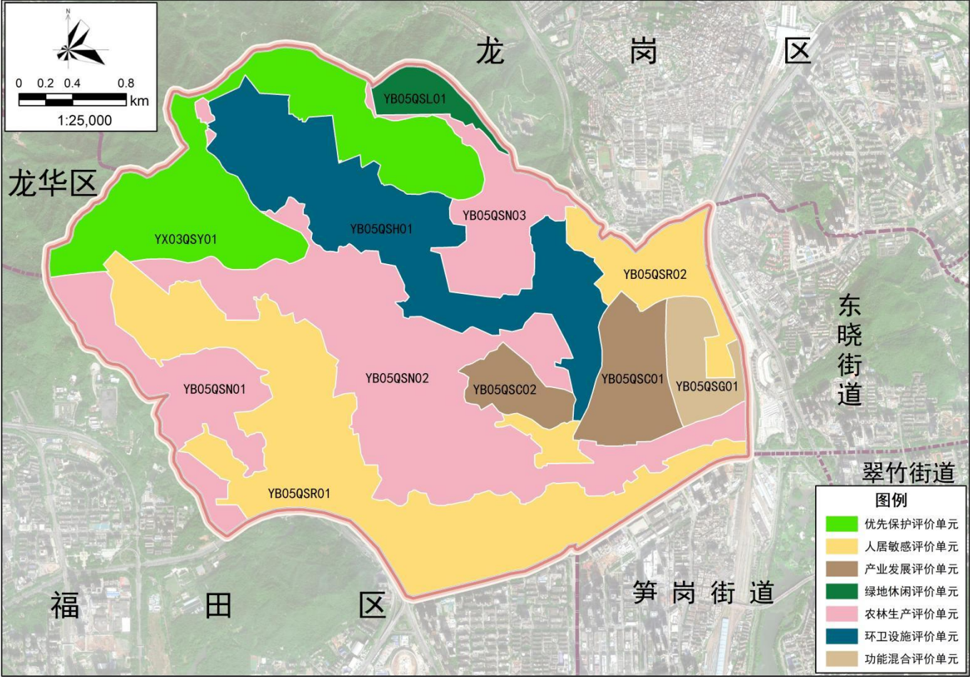
附件 1 罗湖区清水河街道区域空间生态环境评价单元图
